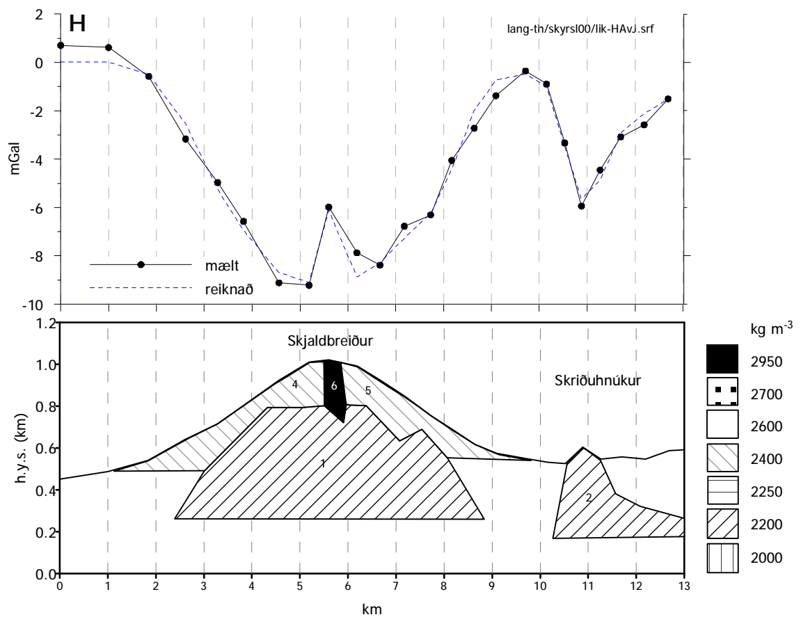
11. mynd. Líkan eftir sniði H: Skjaldbreiður-Skriðuhnúkur.
